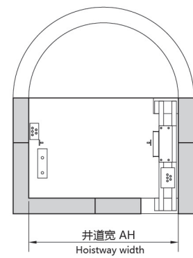
B向 Section B
