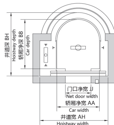
井道布置图 Hoistway plan
